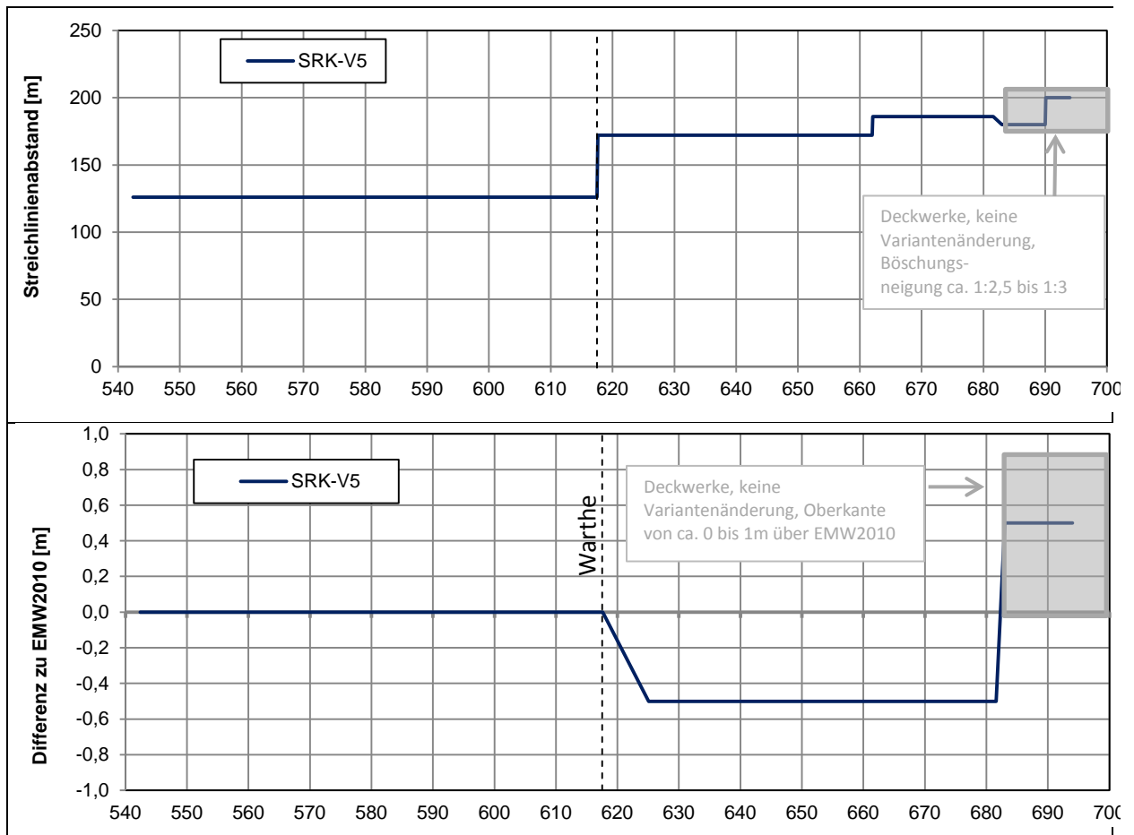
Bild 2-6: Grafik der geometrischen Basisparameter, oben Streichlinienabstände, unten Bauwerkssollhöhe bezogen auf EMW 2010 für Variante SRK-V5
