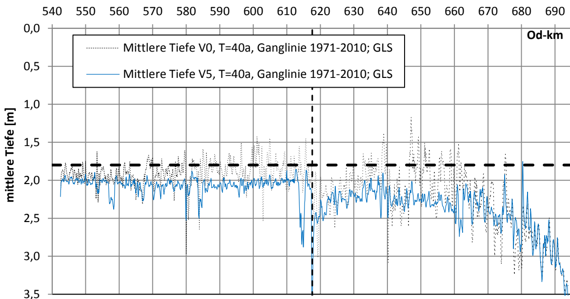
Bild 2-5: Vergleich der mittleren Tiefen bei Q_{P\ddot{U}80/90} der Varianten V0 und SRK-V5 über den gesamten Untersuchungsbereich
