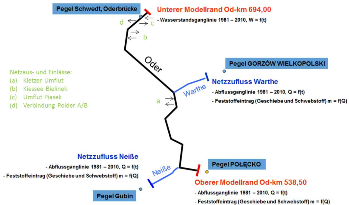
Bild 2-2: Modellnetz, Grenzoder mit Teilstrecken der polnischen Oder, Neiße und Warthe
