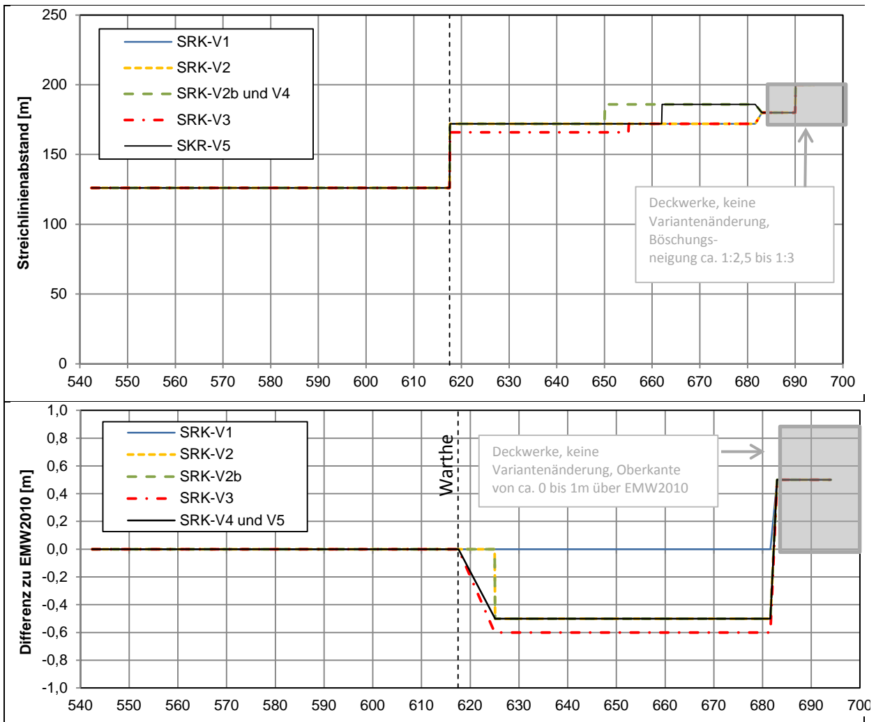
Bild 2-1: Grafische Darstellung der geometrischen Basisparameter, oben Streichlinienabstände, unten Bauwerkssollhöhe bezogen auf EMW 2010
